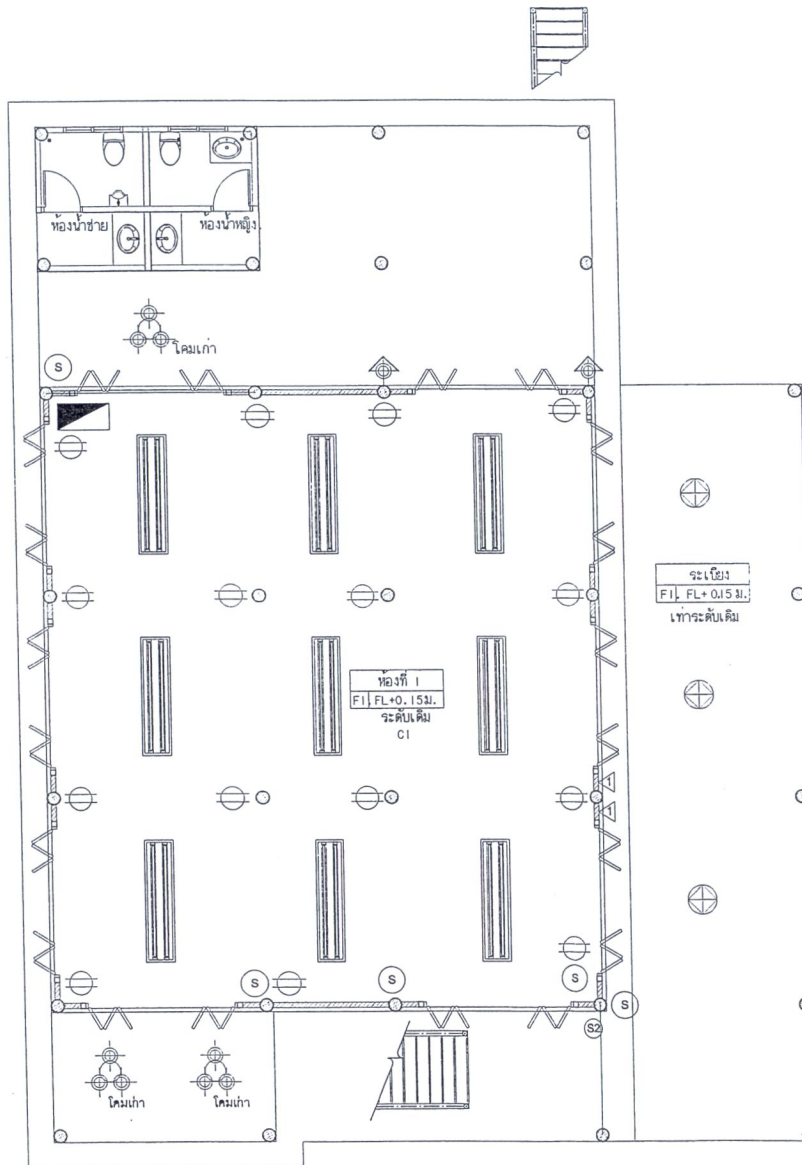
แปลนพื้นไฟฟ้า อาคารหอศิลป์เพื่อการอนุรักษ์ฯ (ปรับปรุง) ชั้น 1 SCALE 1 : 100
